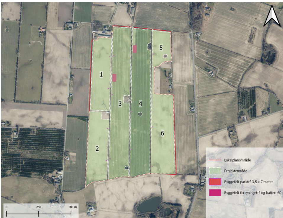
Figur 1. Parklayout for Gudbjerg solcelleprojekt. Layout er foreløbigt, og kan forandres afhængigt af input ifm. miljøvurdering og planfasen.
